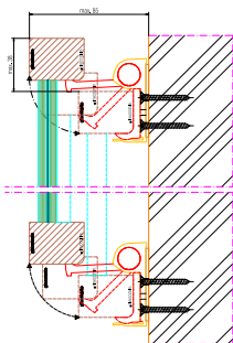
GM WINDOORAIL® profiel hoekig uitgezwenkt
